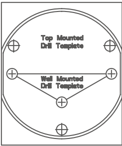
Modelo de perfuração (×1)
